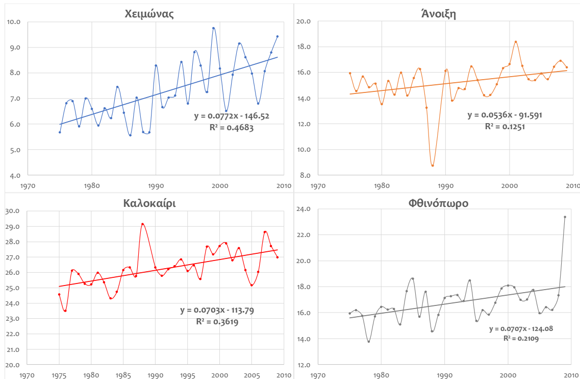
Εικόνα 27: Εποχική διακύμανση της μέσης θερμοκρασίας (οC) στο σταθμό Δράμα για την περίοδο 1975-2009 τον χειμώνα (αριστερά πάνω), την άνοιξη (δεξιά πάνω), το καλοκαίρι (αριστερά κάτω) και το φθινόπωρο (δεξιά κάτω)
