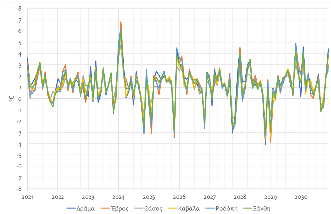
Εικόνα 218: Αποκλίσεις μέσων μηνιαίων τιμών ελάχιστης θερμοκρασίες αέρα στα 2 m (οC) ανά Περιφερειακή Ενότητα την περίοδο 2021-2030 συγκριτικά με την περίοδο 1961-1990 σύμφωνα με τα αποτελέσματα των κλιματικών προσομοιώσεων με το περιοχικό μοντέλο RACMOE2.2. για το Σενάριο RCP4.5.
