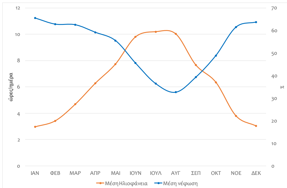
Εικόνα 56: Μηνιαία διακύμανση της μέσης νεφοκάλυψης (%) για το σταθμό Κομοτηνής την περίοδο 1955-2011
