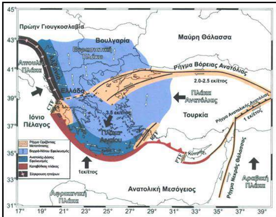
Εικόνα 86: Χάρτης Ανατολικής Μεσογείου της ενεργούς γεωδυναμικής κατάστασης, των κινήσεων των μικροπλάκων και της διαμόρφωσης του Ελληνικού-Αιγαίου τόξου (Παπαζάχος κ.α., 2001)
