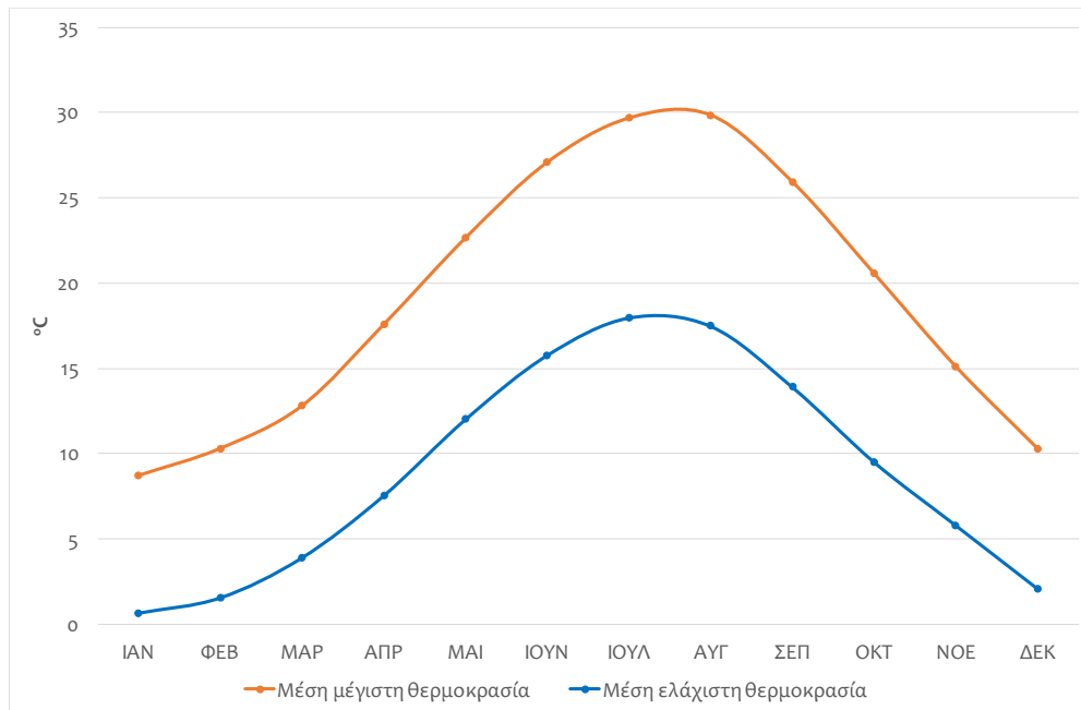
Εικόνα 42: Μηνιαία διακύμανση της ελάχιστης (μπλε γραμμή) και της μέγιστης (πορτοκαλί γραμμή) θερμοκρασίας(°C) για τους σταθμούς Αμυγδαλέωνα την περίοδο 1956-1984 και Χρυσούπολη την περίοδο 1984-2017
