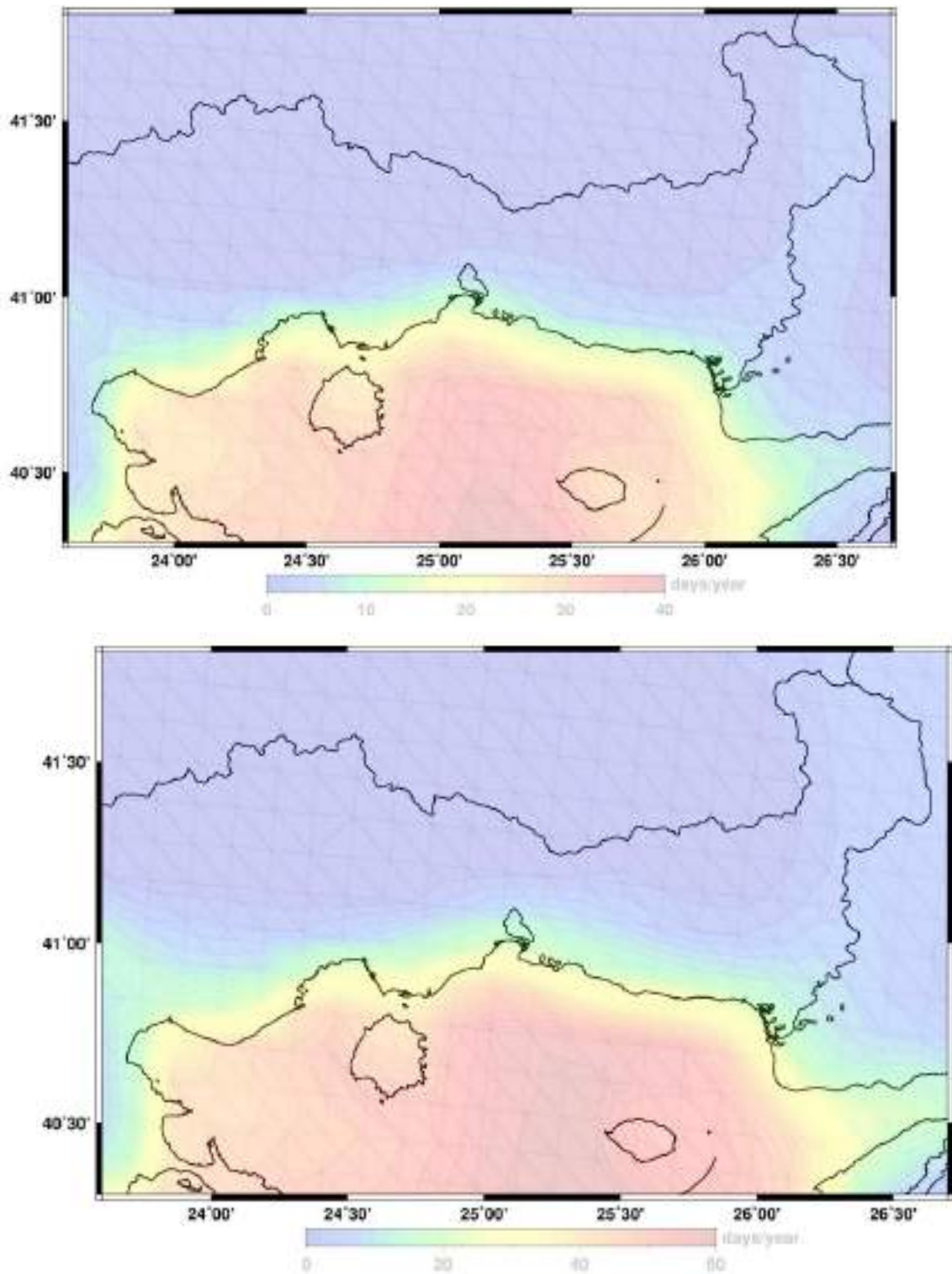
Εικόνα 202: Μεταβολές του αριθμού ημερών ανά έτος με ελάχιστη θερμοκρασία μεγαλύτερη από 20οC μεταξύ των περιόδων 2021-2050 και 1961-1990 (πάνω), 2071-2100 και 1961-1990 (κάτω) σύμφωνα με τα αποτελέσματα των κλιματικών προσομοιώσεων με το περιοχικό μοντέλο RACMOE2.2 για το Σενάριο RCP4.5.
