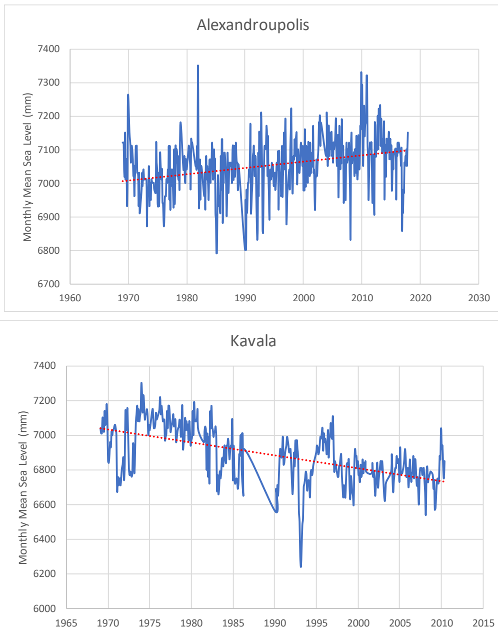
Εικόνα 247: Μέση μηνιαία στάθμη θάλασσας στα σταθμούς σταθμηγράφων του δικτύου της Υδρογραφικής υπηρεσίας του Πολεμικού Ναυτικού στην Αλεξανδρούπολη και την Καβάλα (Πηγή: http://www.psmsl.org/data/obtaining/ )
