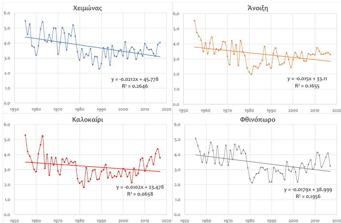
Εικόνα 20: Εποχική διακύμανση της ταχύτητας ανέμου (m/s) στο σταθμό Αλεξανδρούπολη για την περίοδο 1955-2017 τον χειμώνα (αριστερά πάνω), την άνοιξη (δεξιά πάνω), το καλοκαίρι (αριστερά κάτω) και το φθινόπωρο (δεξιά κάτω)
