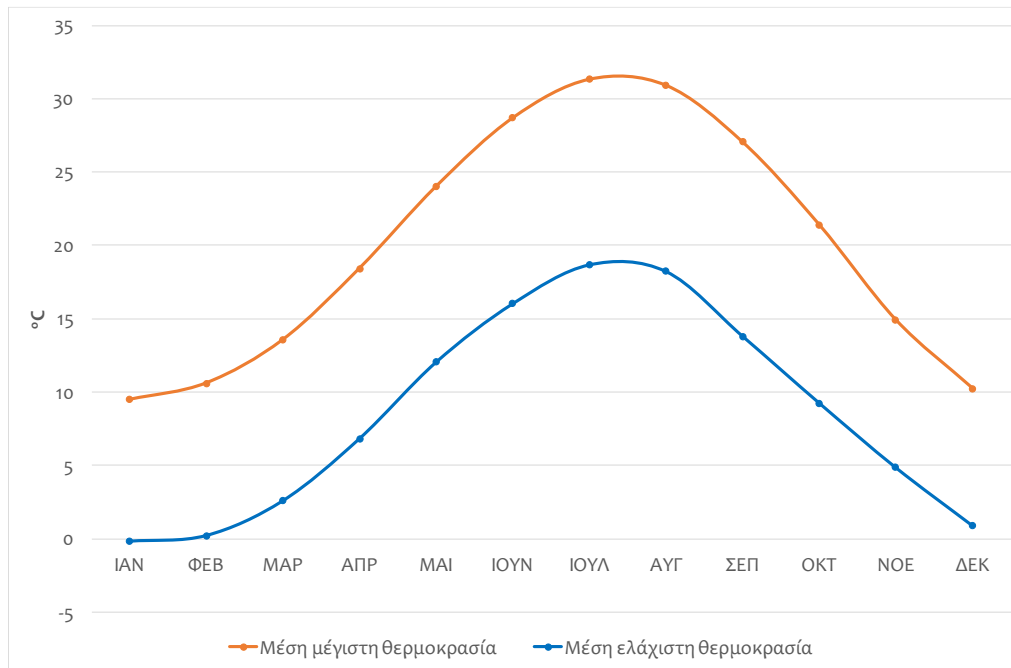
Εικόνα 66: Μηνιαία διακύμανση της ελάχιστης (μπλε γραμμή) και της μέγιστης (πορτοκαλί γραμμή) θερμοκρασίας (°C) για το σταθμό Ξάνθης την περίοδο 1975-2014
