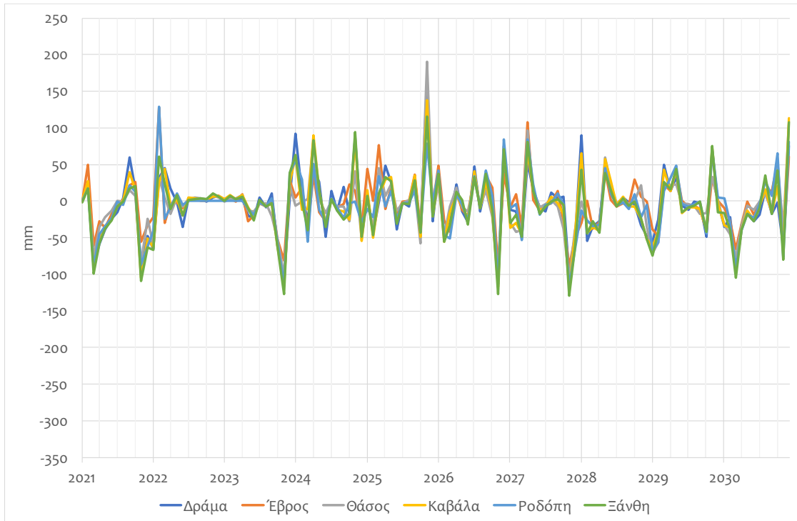
Εικόνα 222: Αποκλίσεις συνολικής μηνιαίας κατακρήμνισης (mm) ανά Περιφερειακή Ενότητα την περίοδο 2021-2030 συγκριτικά με την περίοδο 1961-1990 σύμφωνα με τα αποτελέσματα των κλιματικών προσομοιώσεων με το περιοχικό μοντέλο RACMOE2.2. για το Σενάριο RCP4.5.
