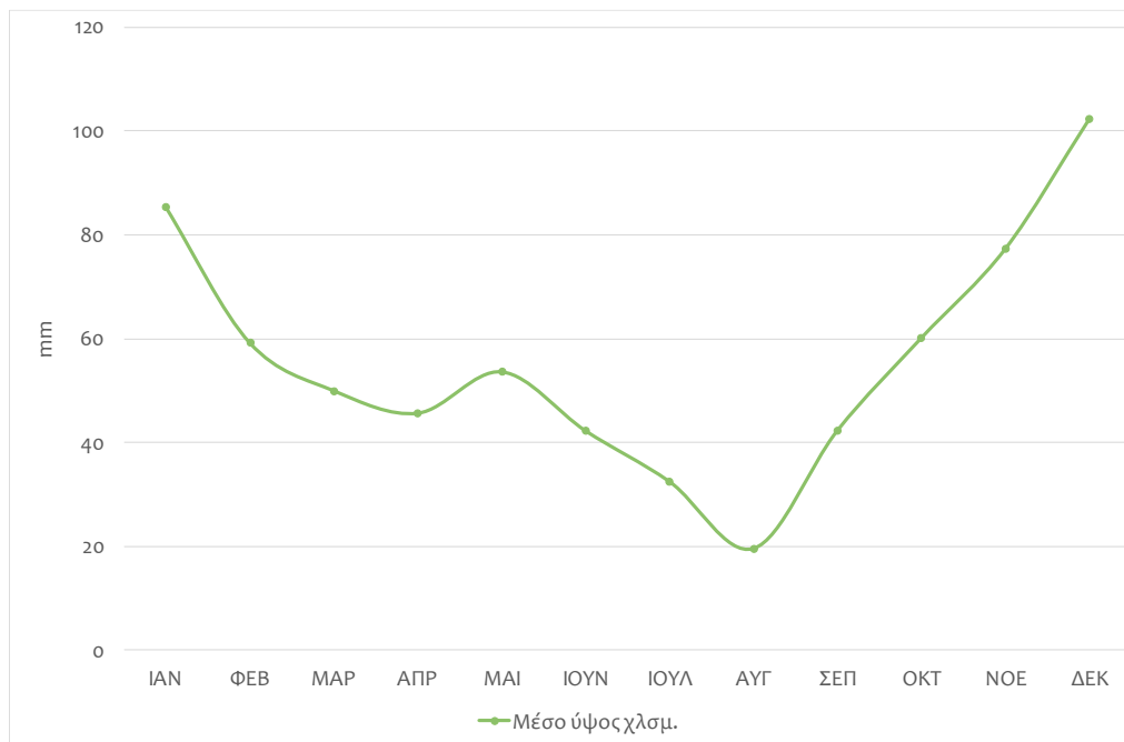
Εικόνα 57: Μηνιαία διακύμανση του μέσου ύψους νετού (mm) για το σταθμό Κομοτηνής την περίοδο 1955-2011
