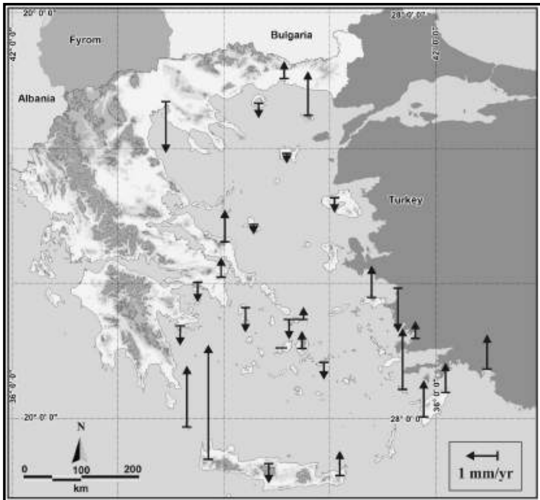
Εικόνα 88: Χωρική κατανομή κινήσεων Τεκτονικής Ανύψωσης (↑) – Καταβύθισης (↓) παράκτιων περιοχών (Pavlopoulos et al., 2011)
