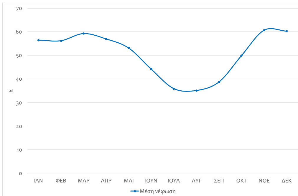
Εικόνα 67: Μηνιαία διακύμανση της μέσης νεφοκάλυψης σε % (μπλε γραμμή) και της μέσης ηλιοφάνειας σε ώρες/ημέρα (πορτοκαλί γραμμή) για το σταθμό Ξάνθης την περίοδο 1975-2014
