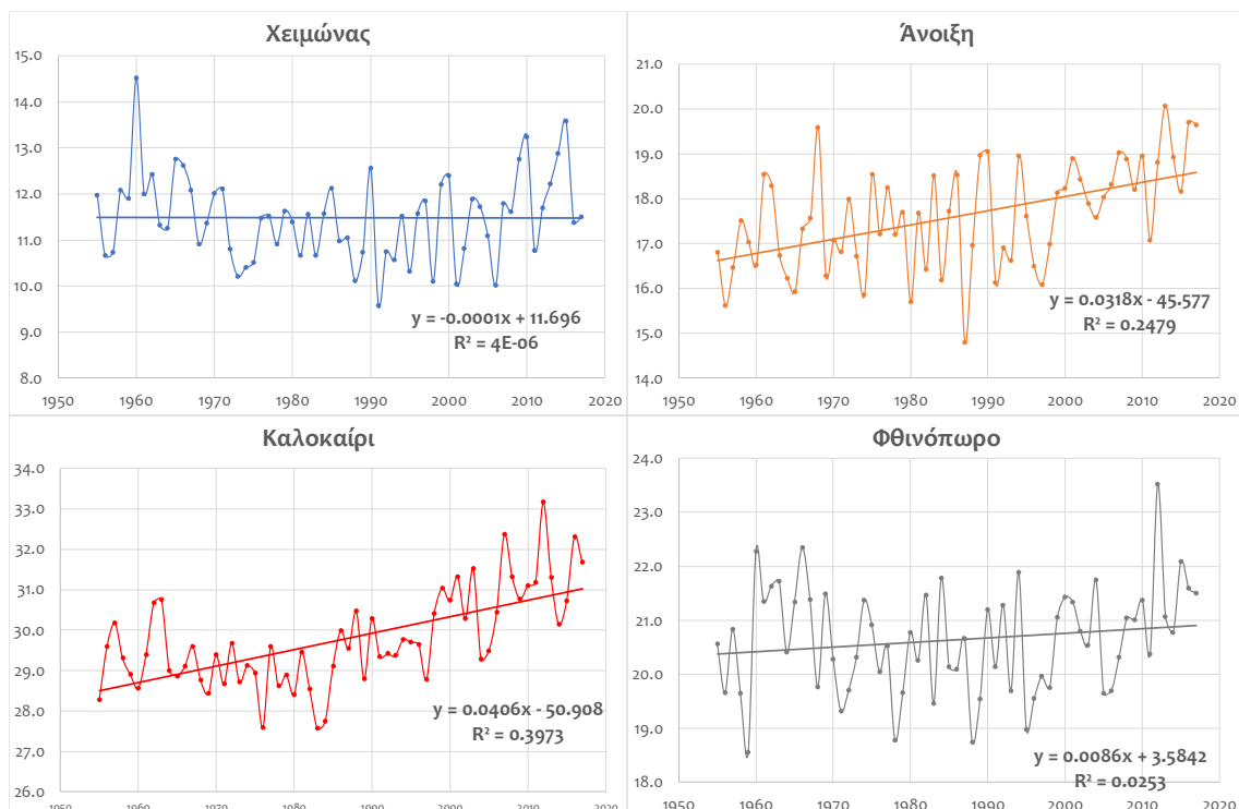
Εικόνα 17: Εποχική διακύμανση της μέσης μέγιστης θερμοκρασίας (°C) στο σταθμό Αλεξανδρούπολη για την περίοδο 1955-2017 τον χειμώνα (αριστερά πάνω), την άνοιξη (δεξιά πάνω), το καλοκαίρι (αριστερά κάτω) και το φθινόπωρο (δεξιά κάτω)
