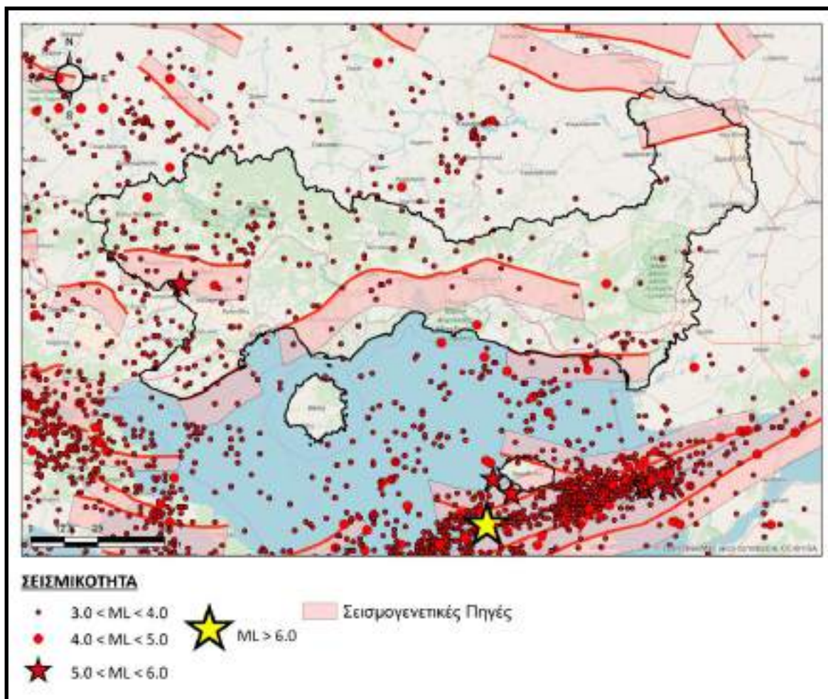
Εικόνα 90: Χάρτης Σεισμικότητας ευρύτερης περιοχής Περιφέρειας Ανατολικής Μακεδονίας και Θράκης (GREDASS, 20014 & Γεωδυναμικό Ινστιτούτο, 2017)
