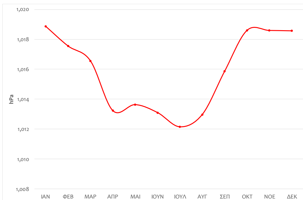
Εικόνα 43: Μηνιαία διακύμανση της ατμοσφαιρικής πίεσης (hPa στην επιφάνεια της θάλασσας) για τους σταθμούς Αμυγδαλέωνα την περίοδο 1956-1984 και Χρυσούπολη την περίοδο 1984-2017
