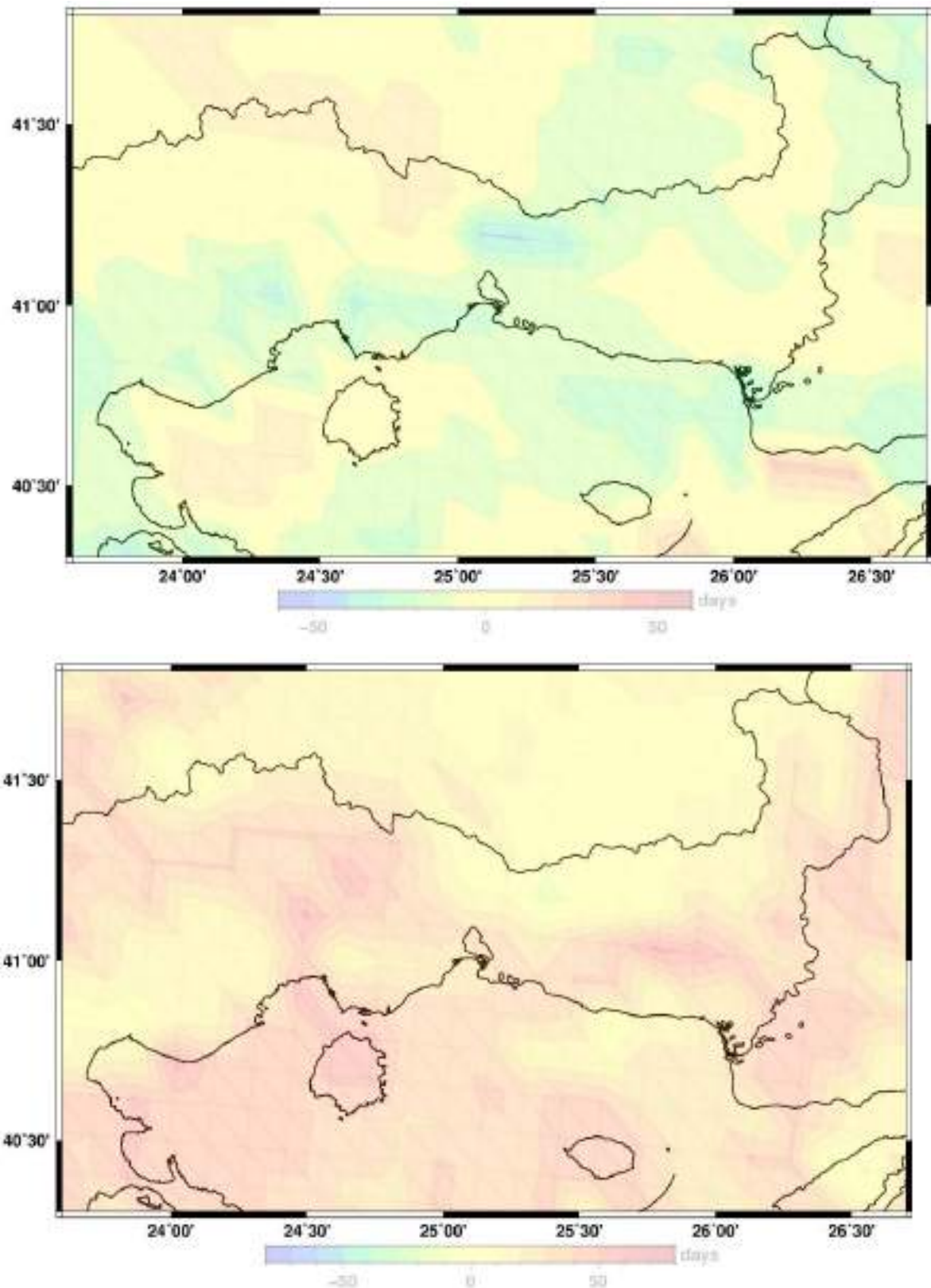
Εικόνα 207: Μεταβολές της μέγιστης διάρκειας ξηρής περιόδου σε ημέρες μεταξύ των ετών 2021-2050 και 1961-1990 (πάνω), 2071-2100 και 1961-1990 (κάτω) σύμφωνα με τα αποτελέσματα των κλιματικών προσομοιώσεων με το περιοχικό μοντέλο RACMO2.2 για το Σενάριο RCP8.5.
