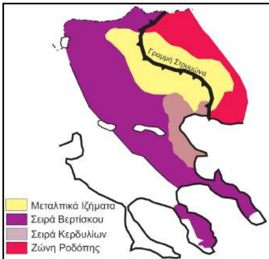
Εικόνα 83: Τεκτονική σχέση Σειράς Βερτίσκου, Κερδυλίων, Ροδόπης και Μεταλπικών Ιζημάτων (Mountrakis et al. 1983)
