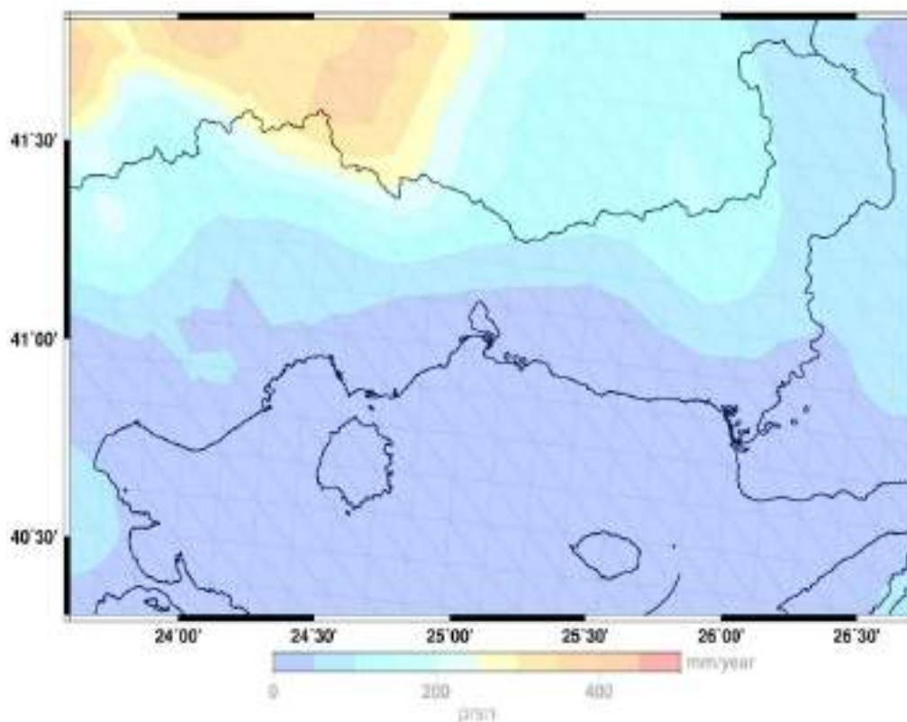
Εικόνα 177: Μέση ετήσια χιονόπτωση (mm) την περίοδο 1961-1990 σύμφωνα με τα αποτελέσματα των κλιματικών προσομοιώσεων με το περιοχικό μοντέλο RACMO2.2.
