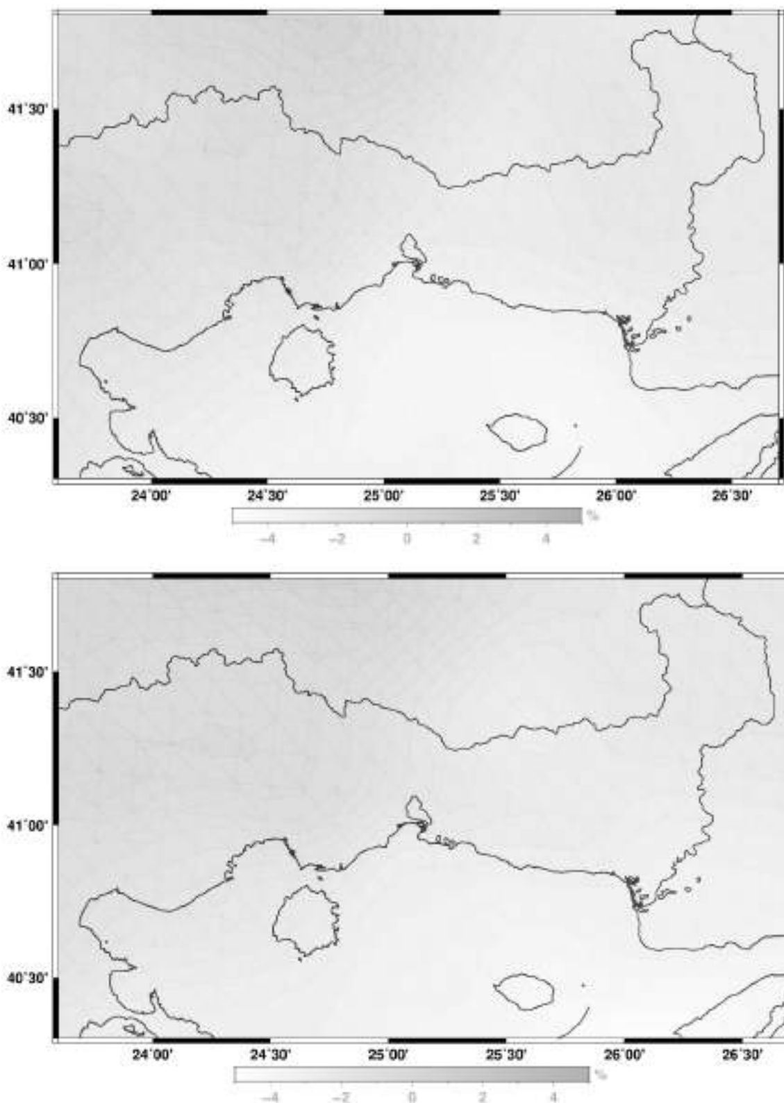
Εικόνα 192: Εκατοστιαίες μεταβολές του μέσου κλάσματος νεφοκάλυψης μεταξύ των περιόδων 2021-2050 και 1961-1990 (πάνω), 2071-2100 και 1961-1990 (κάτω) σύμφωνα με τα αποτελέσματα των κλιματικών προσομοιώσεων με το περιοχικό μοντέλο RACMOE2.2 για το Σενάριο RCP4.5
